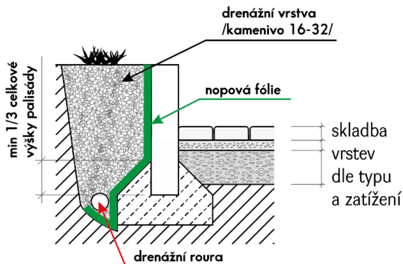
Obr. č.7 Uložení palisád do betonového lože
