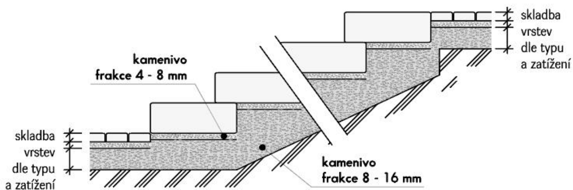
Obr. č. 3 – Uložení do štěrkové lože
