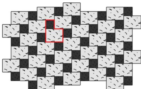
Obr. č.15 – Návrh pokládky z prvků Retro dlažba III. a Retro dlažba I.
