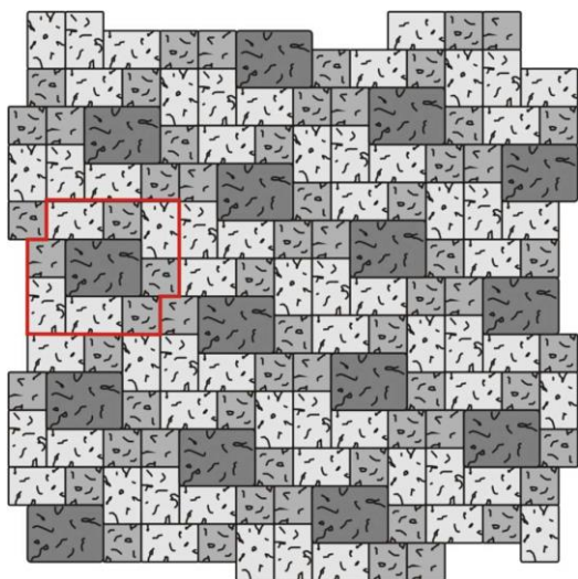
Obr. č.21 – Návrh pokládky z prvků Retro dlažba I., Retro dlažba II. a Retro dlažba III.
