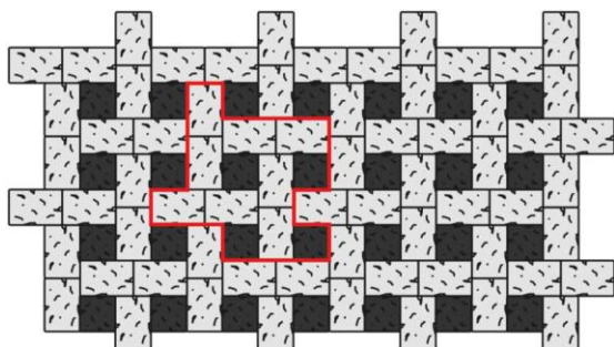
Obr. č.17 – Návrh pokládky z prvků Retro dlažba I. a Retro dlažba II.
