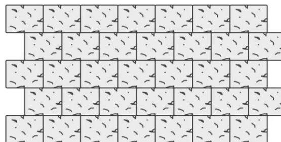
Obr. č.6 – Návrh pokládky z prvků Retro dlažba III.
