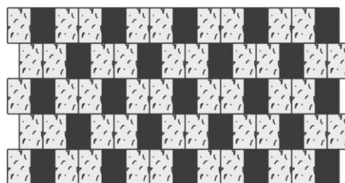
Obr. č.14 – Návrh pokládky z prvků Retro dlažba II.
