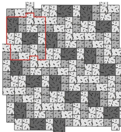
Obr. č.22 – Návrh pokládky z prvků Retro dlažba I., Retro dlažba II. a Retro dlažba III.
