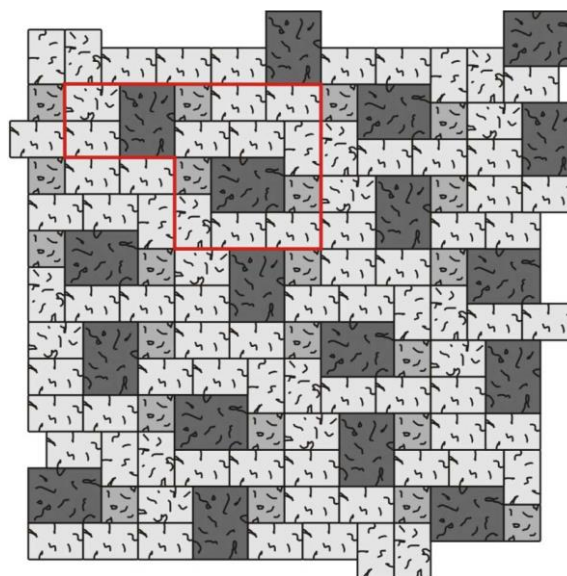
Obr. č.20 – Návrh pokládky z prvků Retro dlažba I., Retro dlažba II. a Retro dlažba III.
