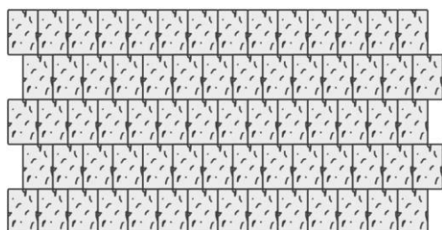
Obr. č.13 – Návrh pokládky z prvků Retro dlažba II.
