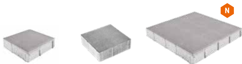
KOCKA 6 Rozmery: 20 × 20 × 6 cm KOCKA 6 ROVNÁ HRANA Rozmery: 20 × 20 × 6 cm KOCKA 8 Rozmery: 20 × 20 × 8 cm KOCKA 8 ROVNÁ HRANA Rozmery: 20 × 20 × 8 cm KOCKA 10 ROVNÁ HRANA Rozmery: 20 × 20 × 10 cm
