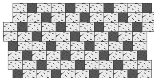
Obr. č.16 – Návrh pokládky z prvků Obdélník 21 / 14 / 7 History a Čtverec 14 / 14 / 7 History
