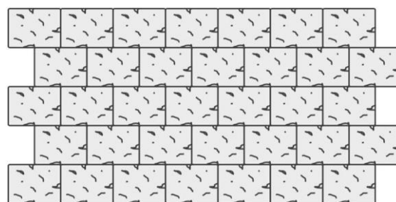
Obr. č.6 – Návrh pokládky z prvků Obdélník 28 / 21 / 7 History
