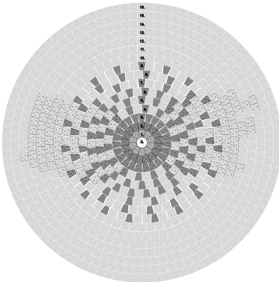
Obr. č.23 – Návrh pokládky do kruhu z prvků K0, K1, K2 a Čtverec 14 / 14 / 7
