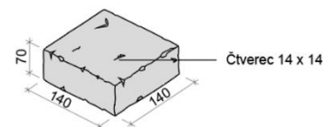
Obr. č.23 – Rozměry kamenů K0, K1, K2 a Čtverec 14 / 14 / 7
