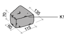
Obr. č.23 – Rozměry kamenů K0, K1, K2 a Čtverec 14 / 14 / 7
